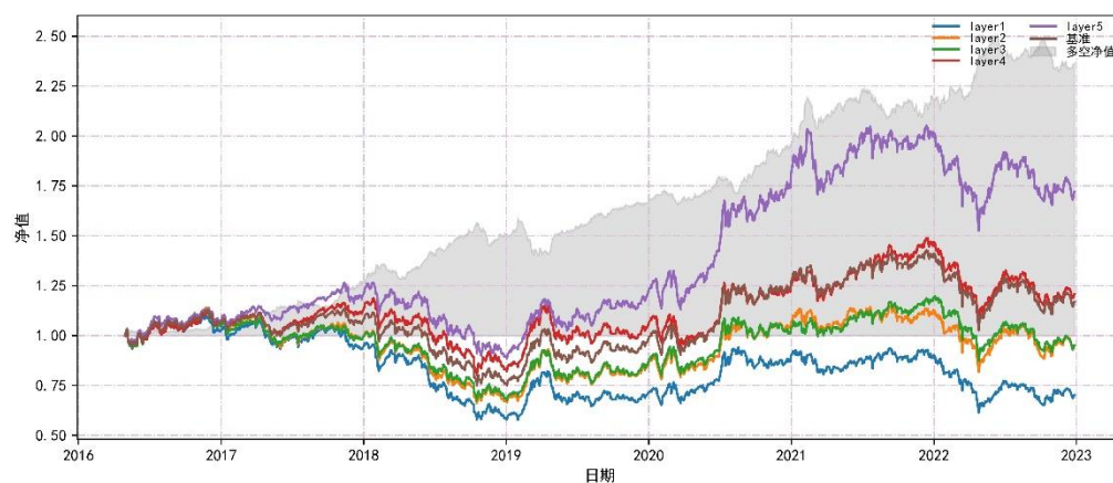
图 13: ABCFO_Q4 在全 A 中的分组效果 (交易费用: 双边千三)
