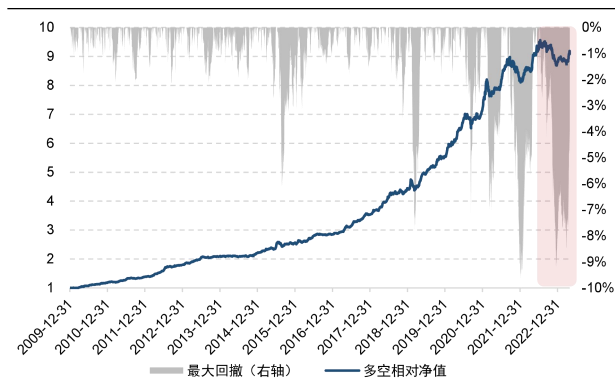
图2：净利润增速因子多空净值及最大回撤
