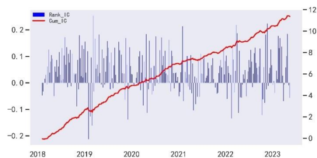
图 76: UOidr Rank IC 表现 (中证 500)
