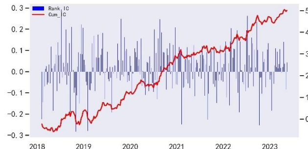
图 68: UOIDR Rank IC 表现（沪深 300）
