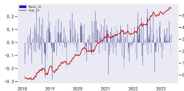
图 70: ID_VOV Rank IC 表现 (沪深 300)
