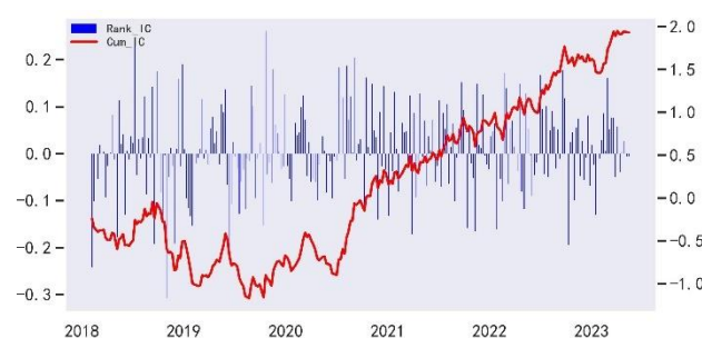
图 72: ID_VOcVaR95 Rank IC 表现 (沪深 300)
