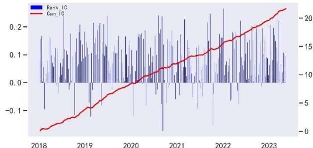
图 32: ID_cVaR95_RT_week 因子 Rank IC 表现
