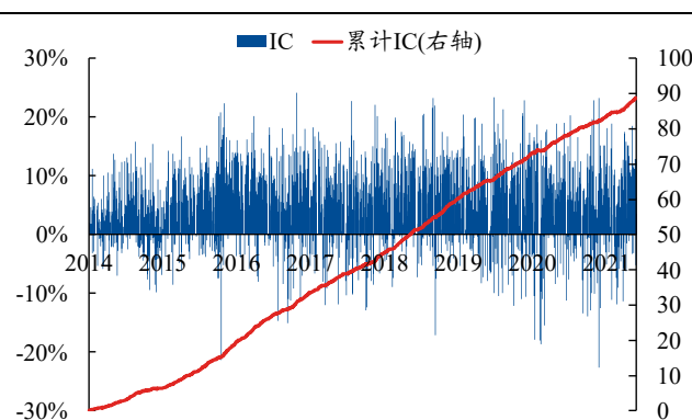
图 21、gmm_meandif2wgtdif 因子 IC 与累计 IC
